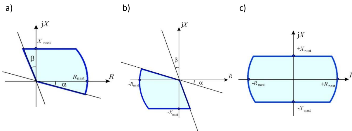
Rys. 15.4.2. Charakterystyki zabezpieczenia podimpedancyjnego w zespołach extCZIP: a) „do przodu”, b) „do tyłu”, c) bezkierunkowa.
