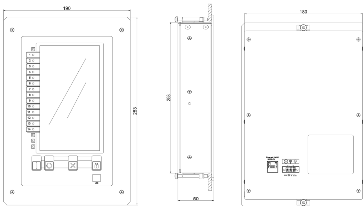
Wymiary otworu w płycie montażowej
