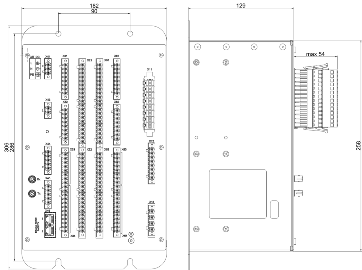
Rys. 7.3 Wersja natablicowa z zewnętrznym panelem operatorskim – jednostka centralna.
