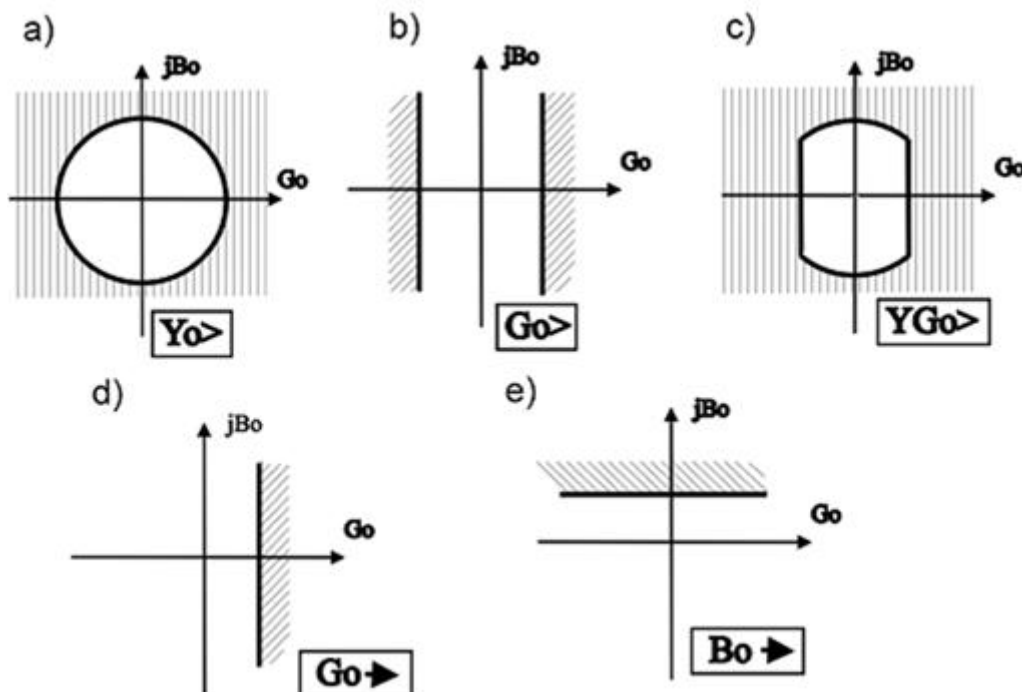
Rys. 15.7.3. Charakterystyki zabezpieczeń ziemnozwarciowych.
