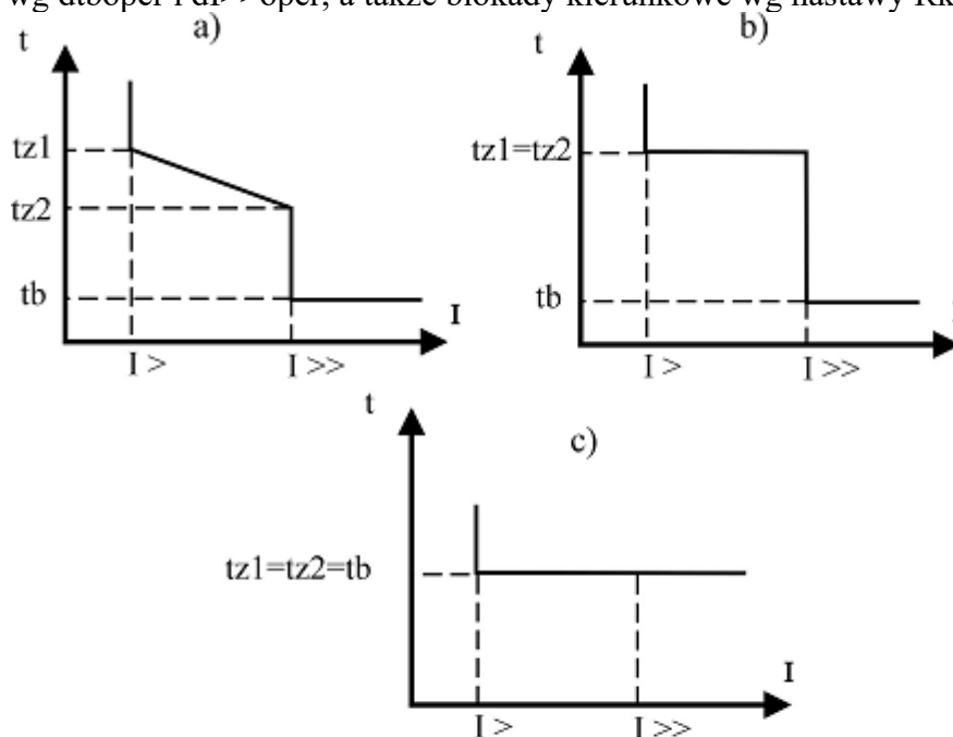
Rys. 15.2.3. Sposób kształtowania charakterystyki czasowej zabezpieczenia od skutków zwarć międzyfazowych: a) łamana, b) dwustopniowa, c) jednostopniowa
